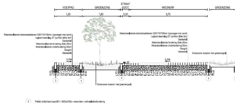
TYPE DWARSPROFIEL A-A schaal 1:50
