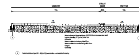
TYPE DWARSPROFIEL G-G
