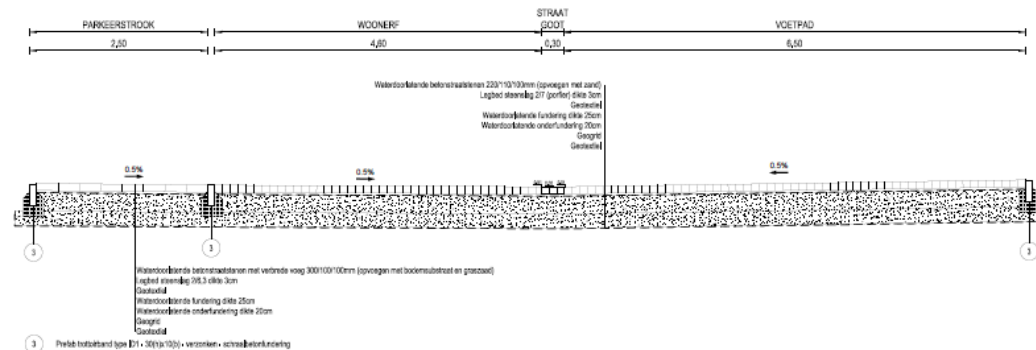
TYPE DWARSPROFIEL B-B
