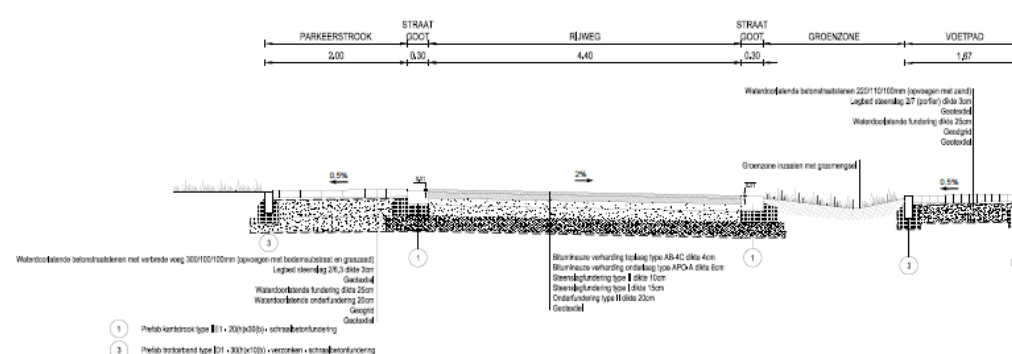
TYPE DWARSPROFIEL D-D schaal 1:50
