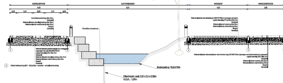
TYPE DWARSPROFIEL F-F
