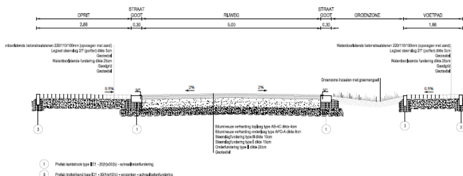
TYPE DWARSPROFIEL C-C schaal 1:50
